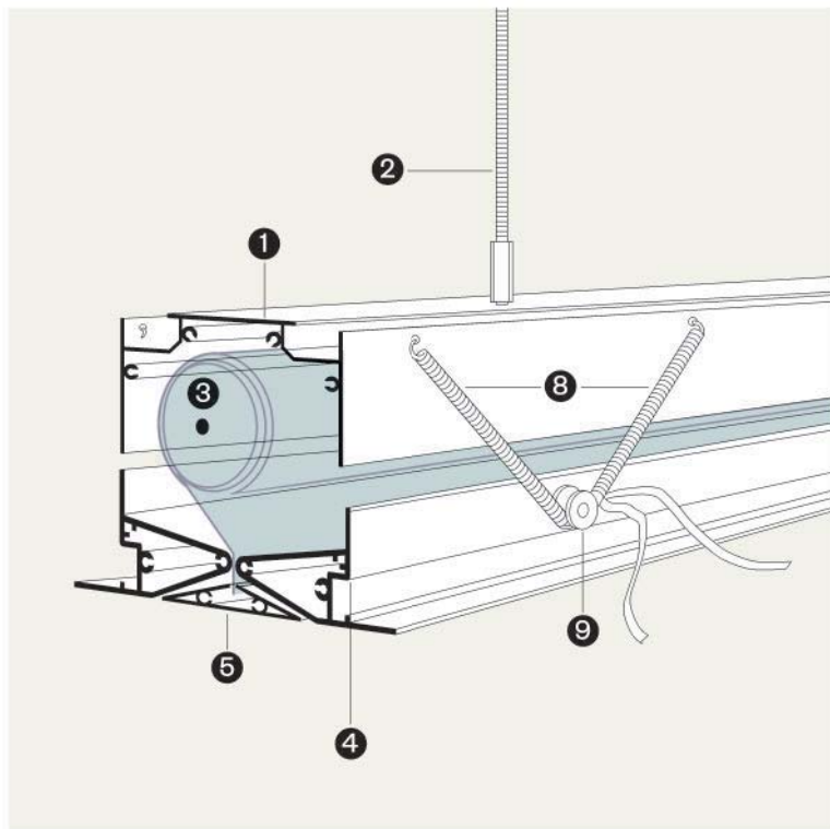
Fissaggio cornice con molla Spring frame fastening 带有弹簧的安装支架 Монтаж системы и внешнего карниза
